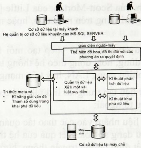
Hình7 . Kiến trúc hệ thống trợ giúp quyết định
