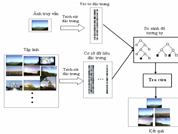
Hình 4.8. Kiến trúc của Module tra cứu group2.
