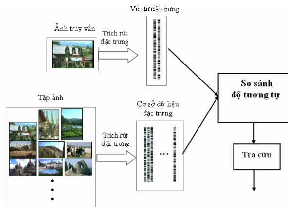
Hình 4.2. Kiến trúc của Module tra cứu group1.
