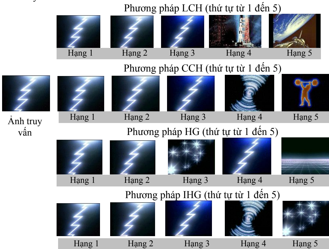
Hình 4.16. Kết quả thực hiện truy vấn 1.
