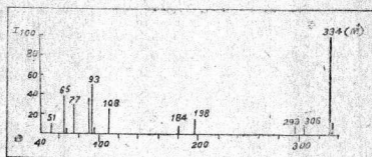
Hình 2: Phổ khối của 1-Phenyl-3-pyrolyl-5-p-nitrophenyl-fomazan
