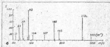
Hình 1: Phổ khối của 1, 3, 5-Triphenylfomazan
